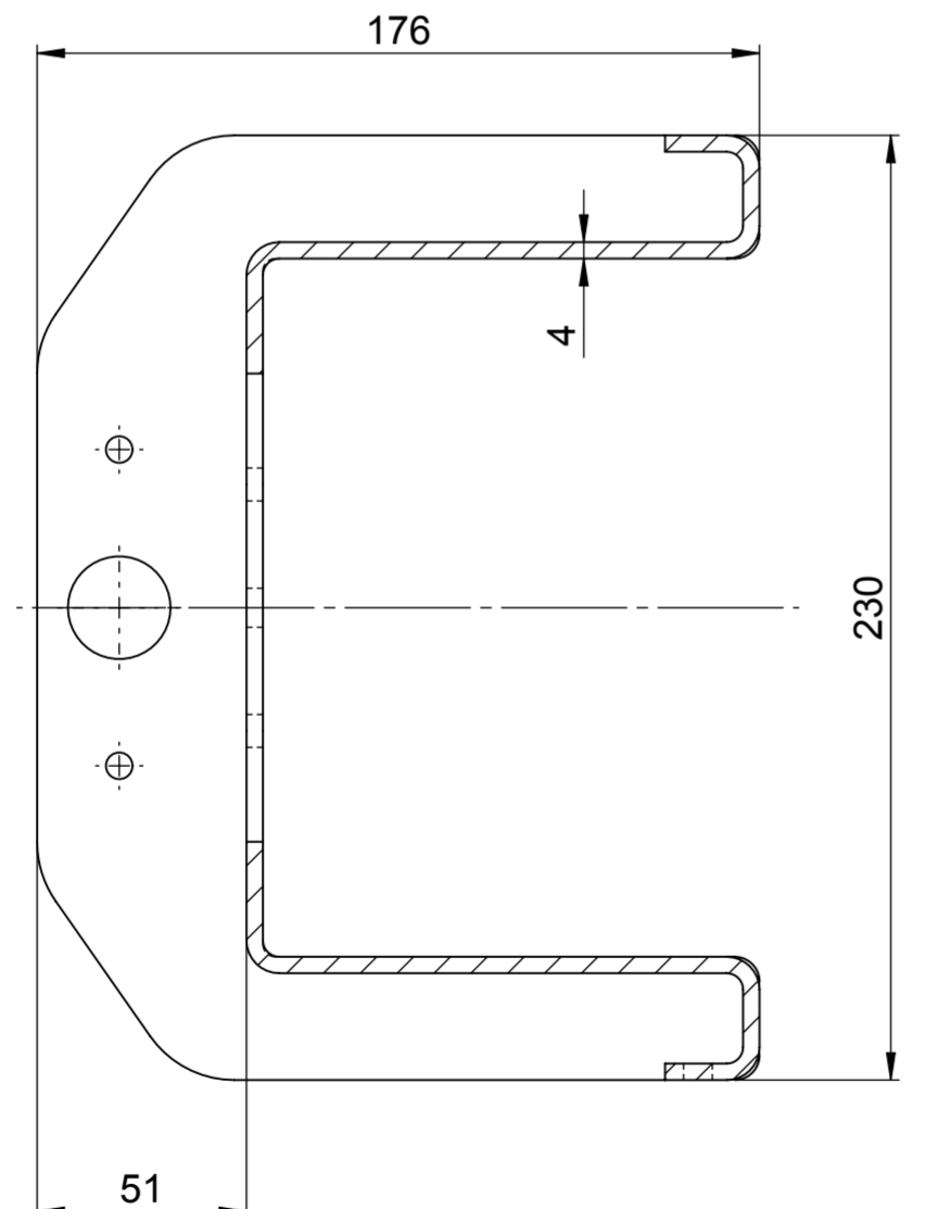
X-X (1 : 2)
